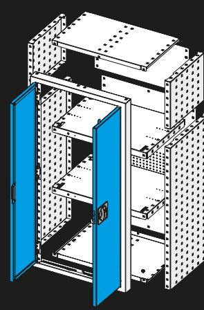
Stepped version for different depths Versión cortada a medida con escalón para cambio profundidad
