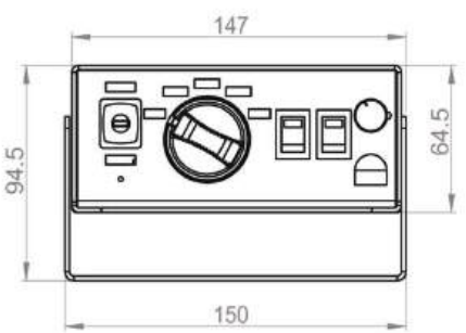
EC-100 & EC-200
