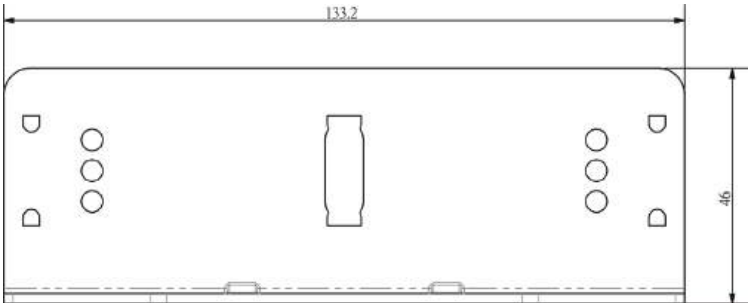
BOLD 12 L-BRACKET
