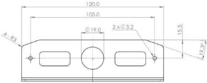
ULTRA-L-BRACKET
