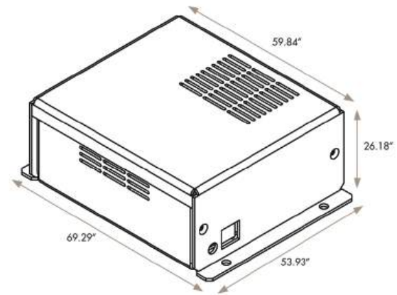
EH-200
